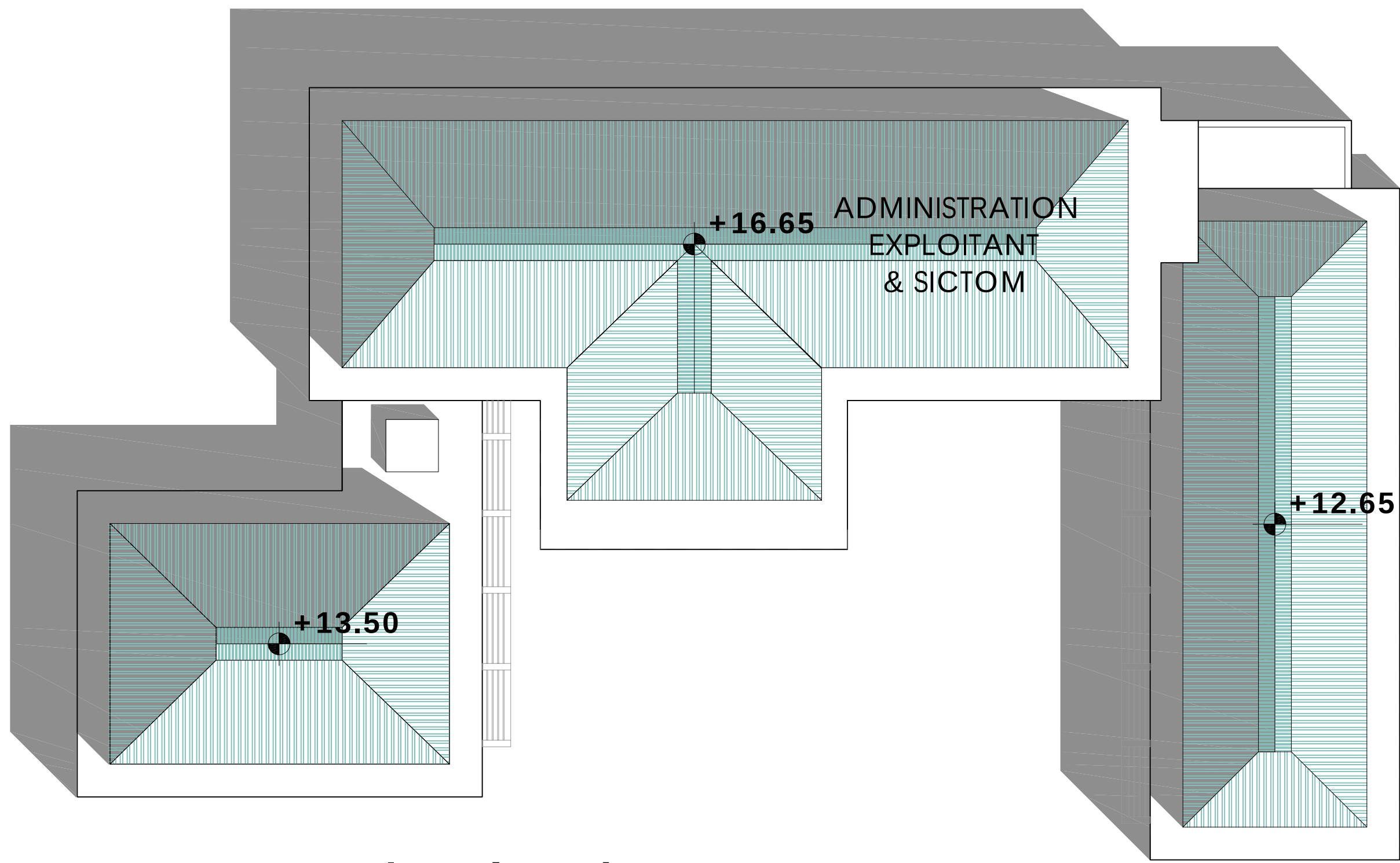
Plan de Toiture
