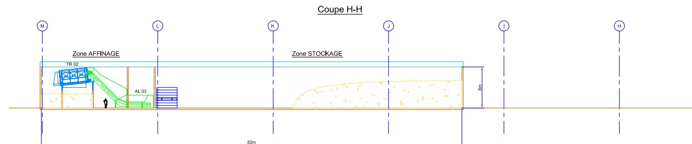
Coupe H-H
