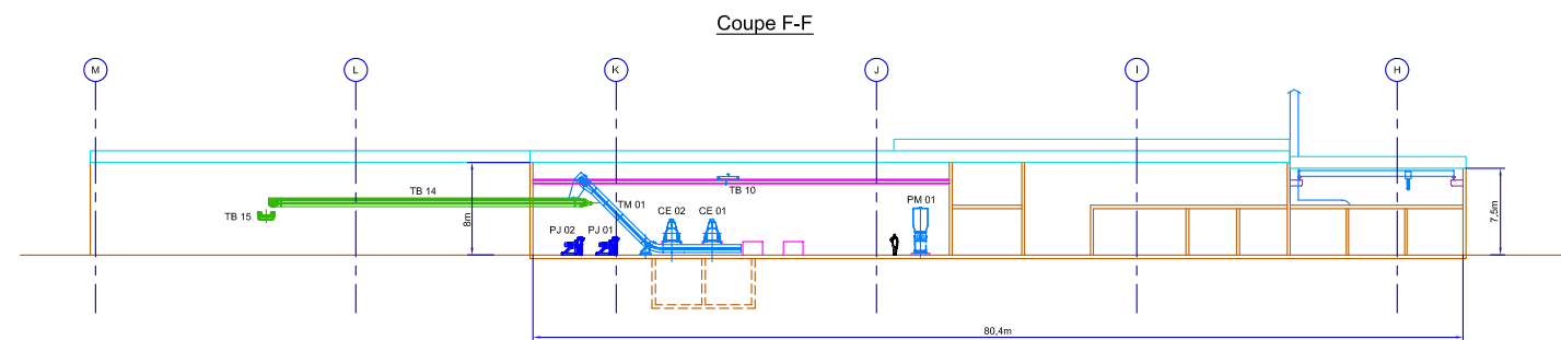
Coupe F-F
