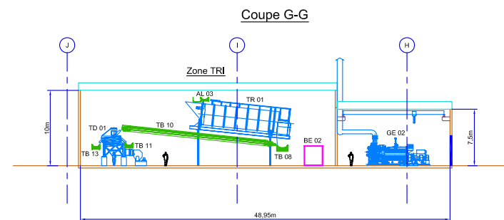
Coupe G-G
