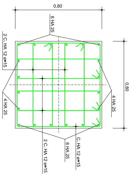
COUPÉ A-A POTEAUX TYPE - 2 ESCALA 1:10
