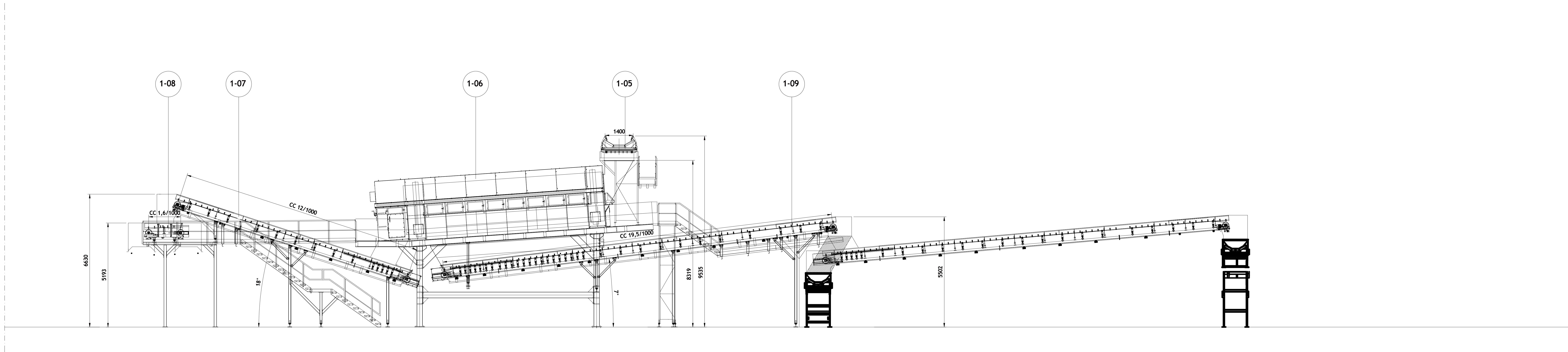
SECCIÓN J-J
