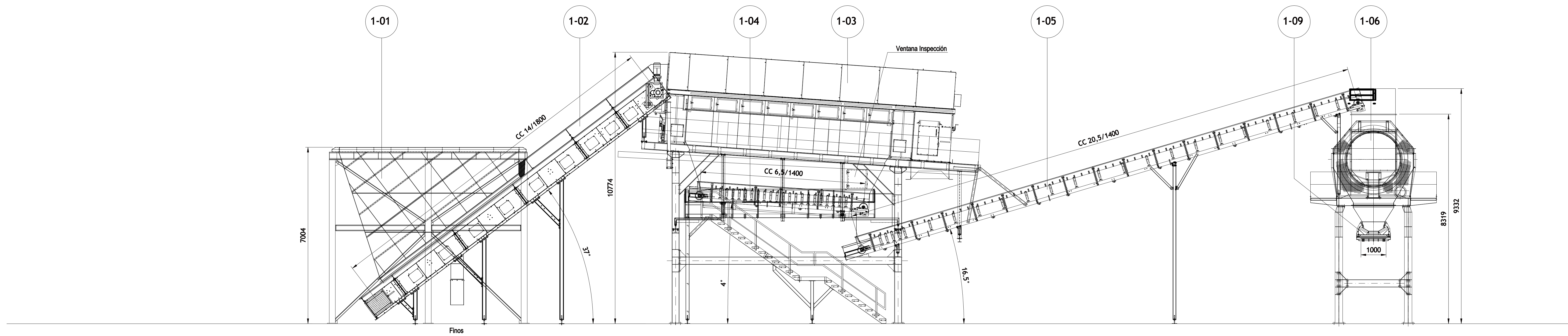
SECCIÓN E-E
