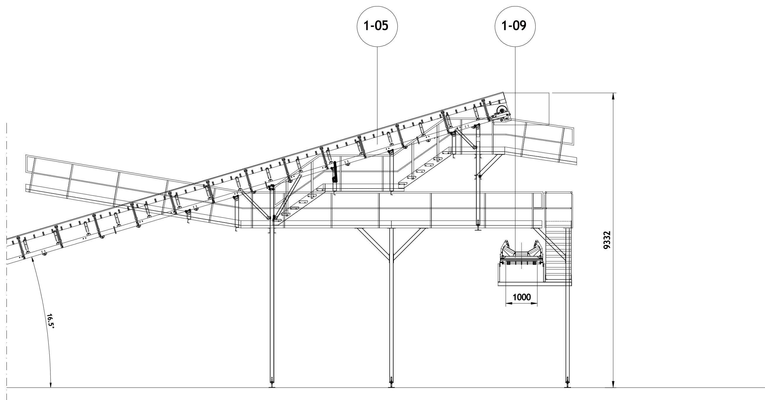
SECCIÓN F-F
